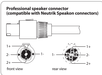
Fig. 4.5: Conector profesional de altavoz con polaridades
