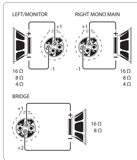
Fig. 4.6: Ocupación de pines (Speakon)
