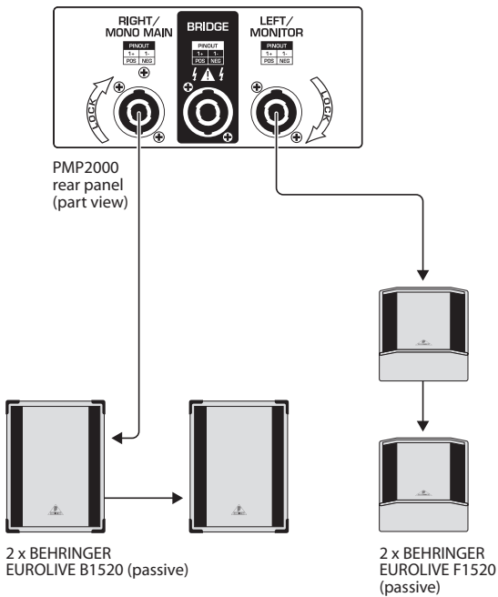
Fig. 5.2: PMP2000 como amplificador doble mono (ejemplo)
